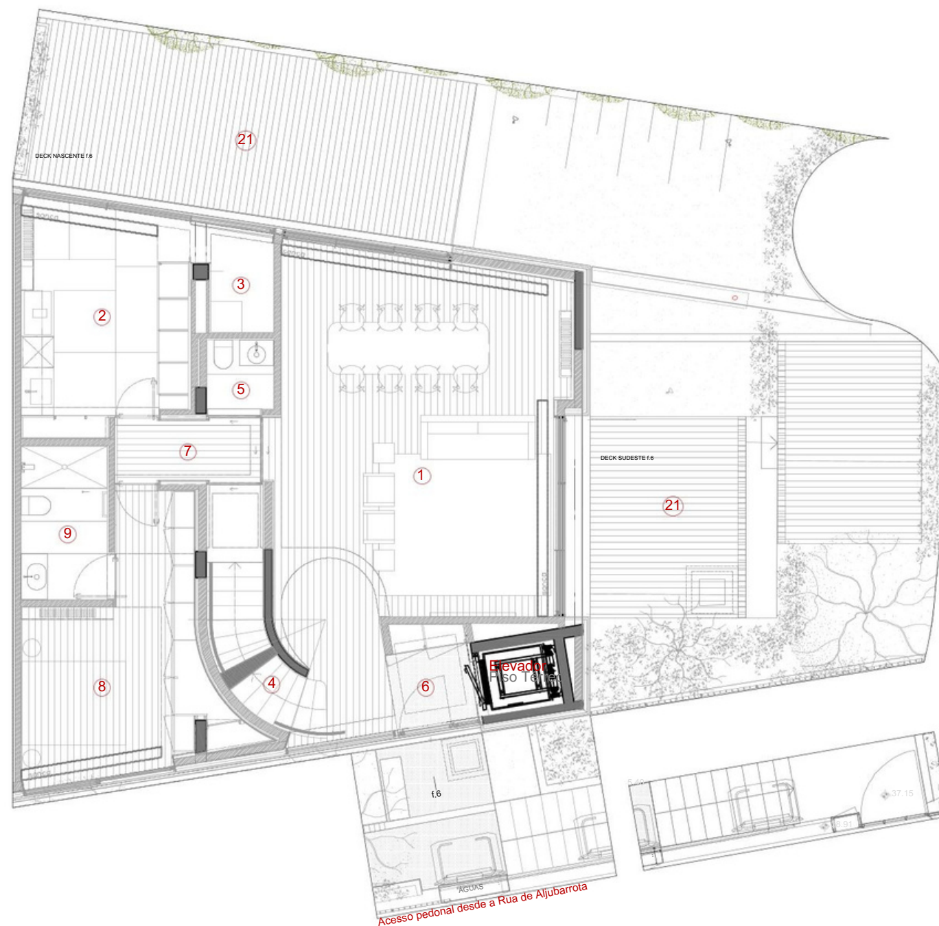
PISO TÉRREO
